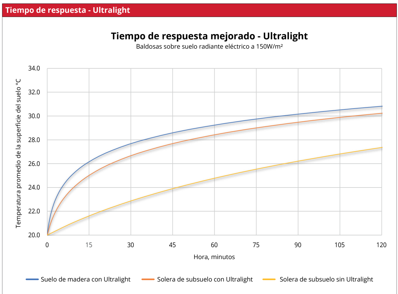
Figura. 2 - Mejora en el tiempo de respuesta debido al uso de Ultralight En las pruebas, con una malla radiante de 150 W / m 2 sobre un solado de 65 mm, el suelo tardará 110 minutos en alcanzar los 27 ° C. Al instalar Ultralight debajo de la calefacción por suelo radiante eléctrica, se alcanza la misma temperatura en solo 34 minutos.
